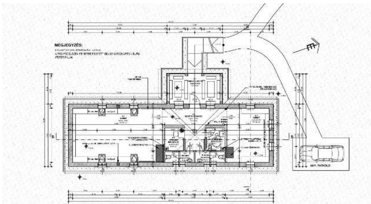
A tervezett épület alaprajza
